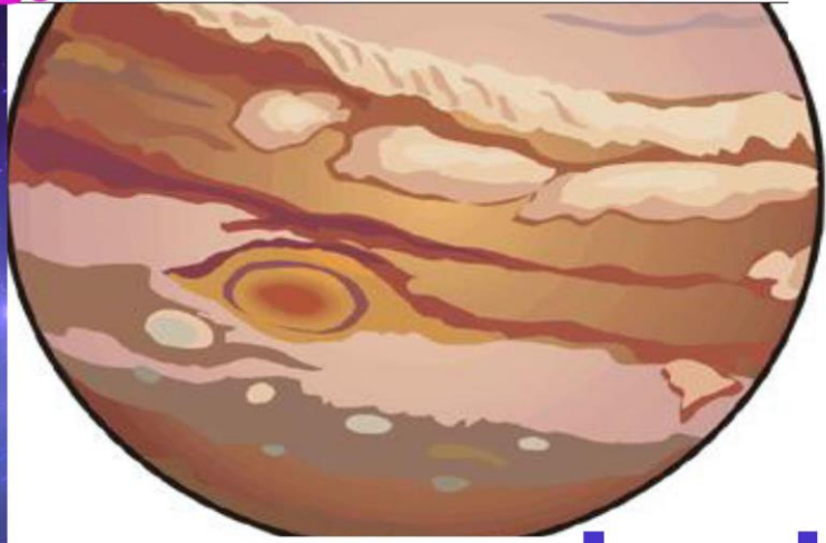
Jupiter
