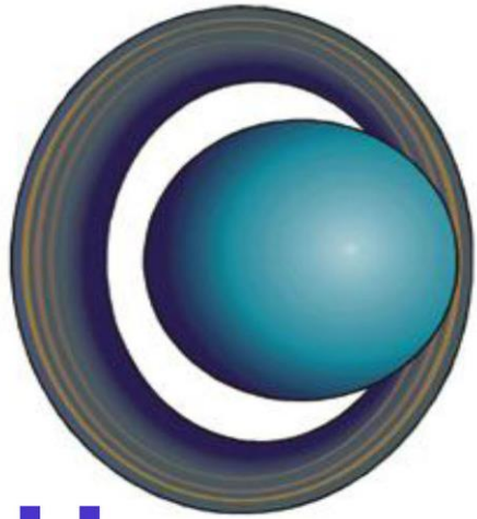
Uranus
