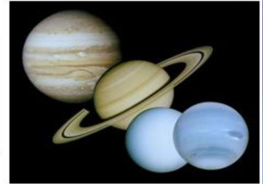
solsystemet
