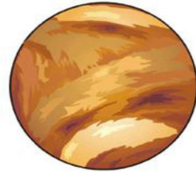
Venus
