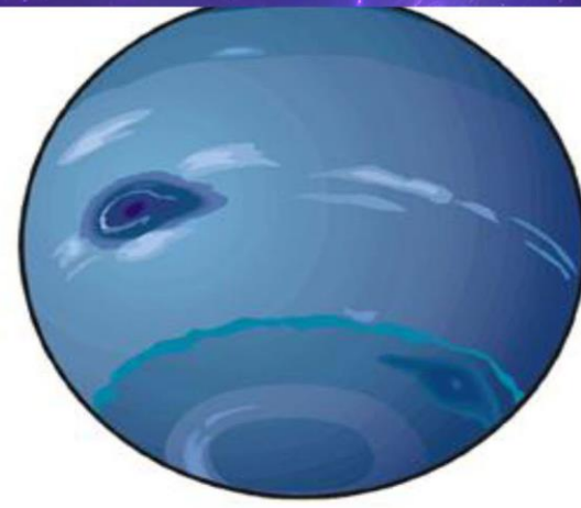
Neptun
