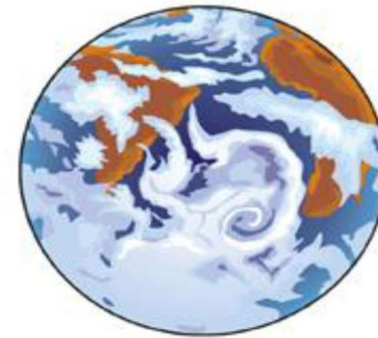
Jorden
